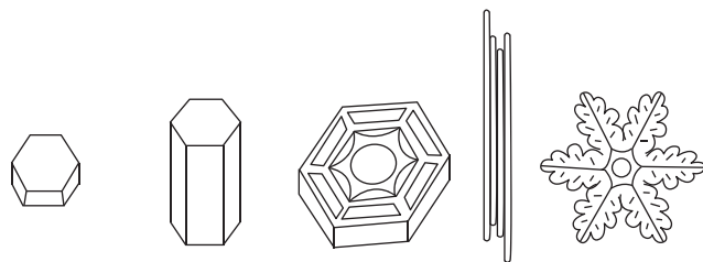
雪晶形态图
